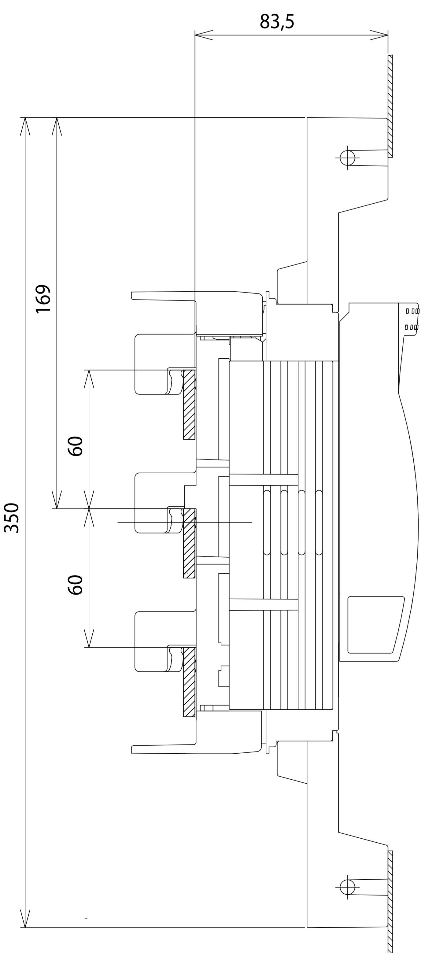
NH-Reiter-LTS Gr.00
