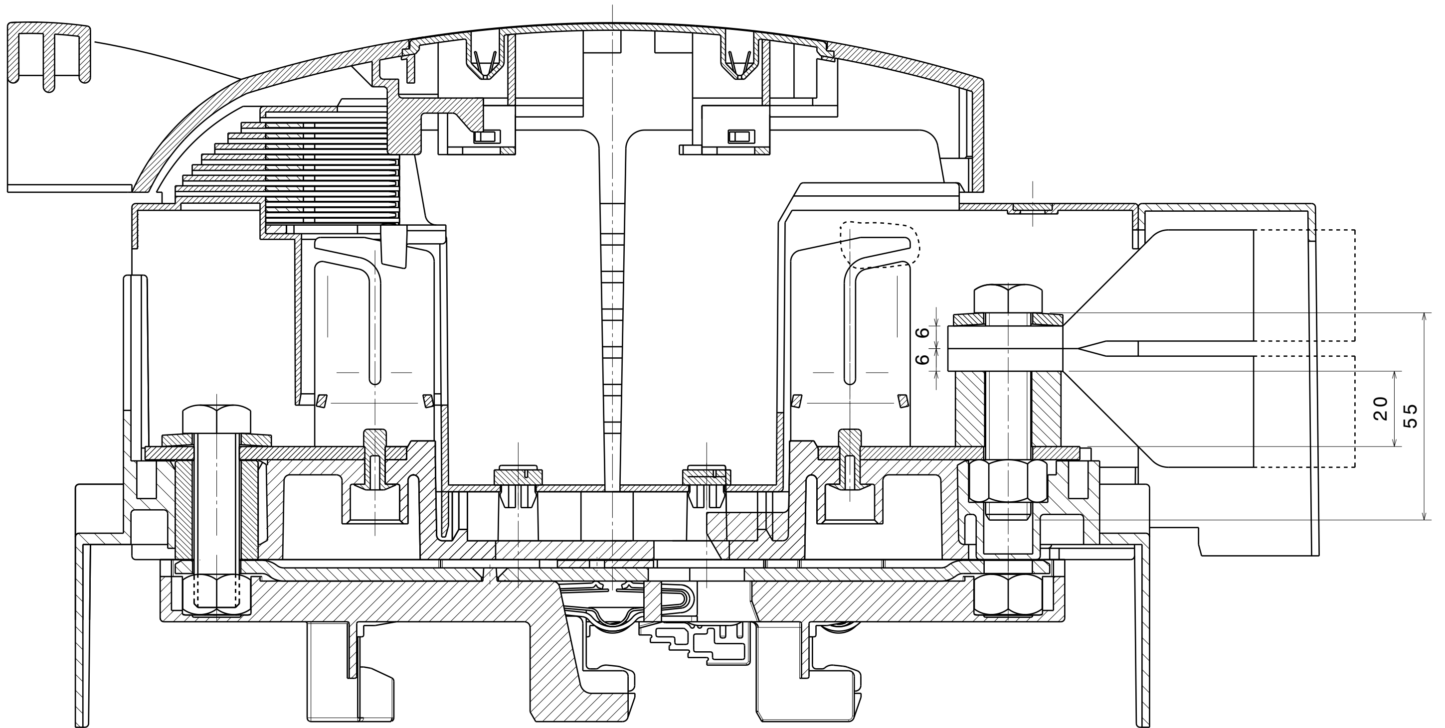
NH-Trenner Gr.3 und 3 x 33 272 zum Anschluss von 2 Kabelschuhen an jeden Kontakt
