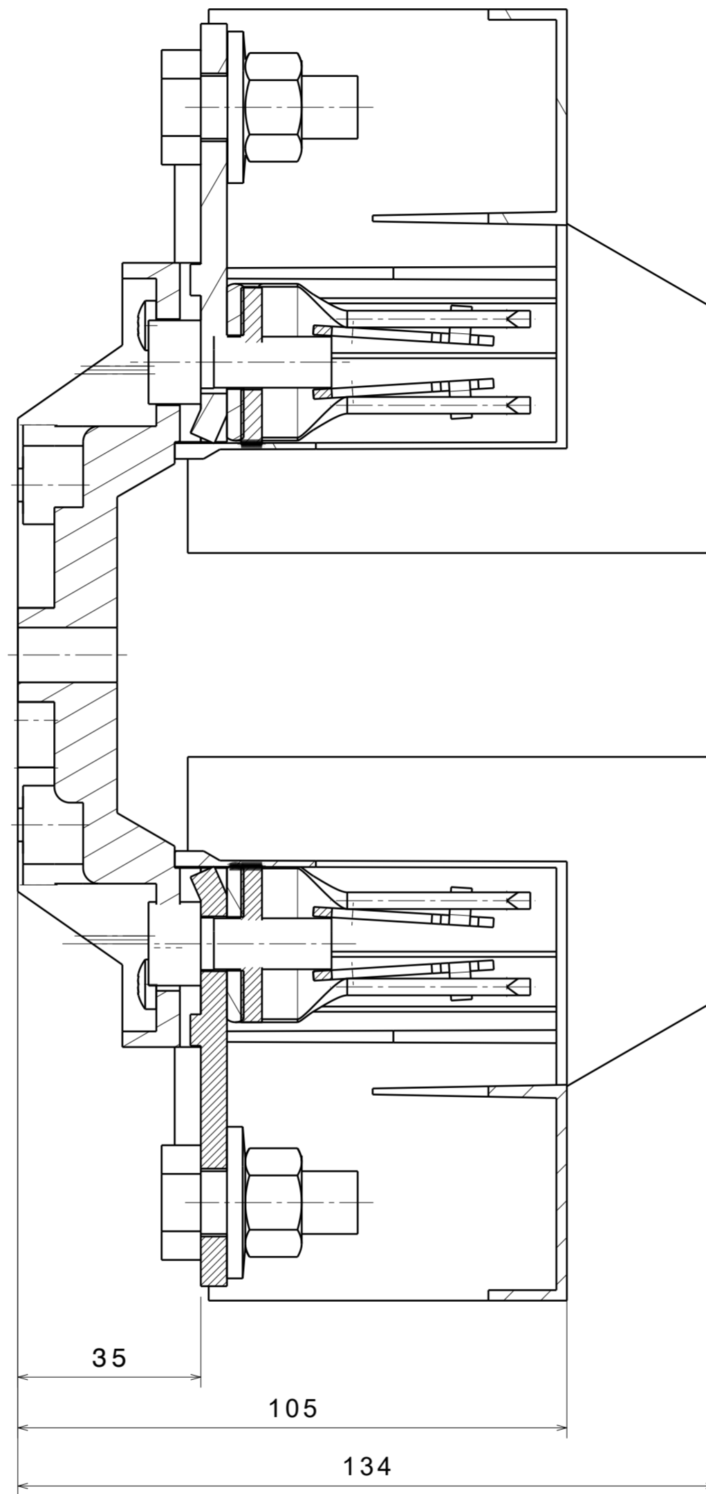
Schnittansicht A-A section view A-A Maßstab: 1:1 scale: 1:1
