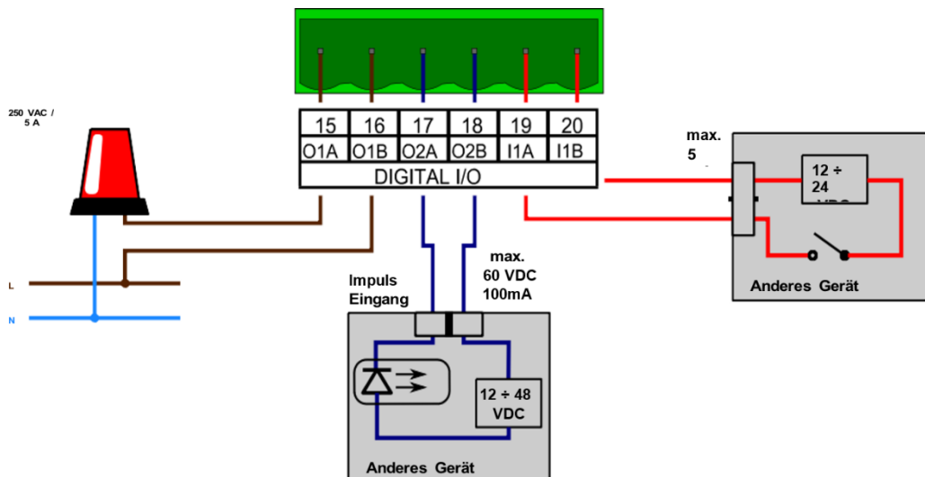
Abbildung 2: Anschlussbeispiel der digitalen Ein-/Ausgänge. Ausgang 1 ist in diesem Beispiel ein Relaisausgang (kein Standard)
