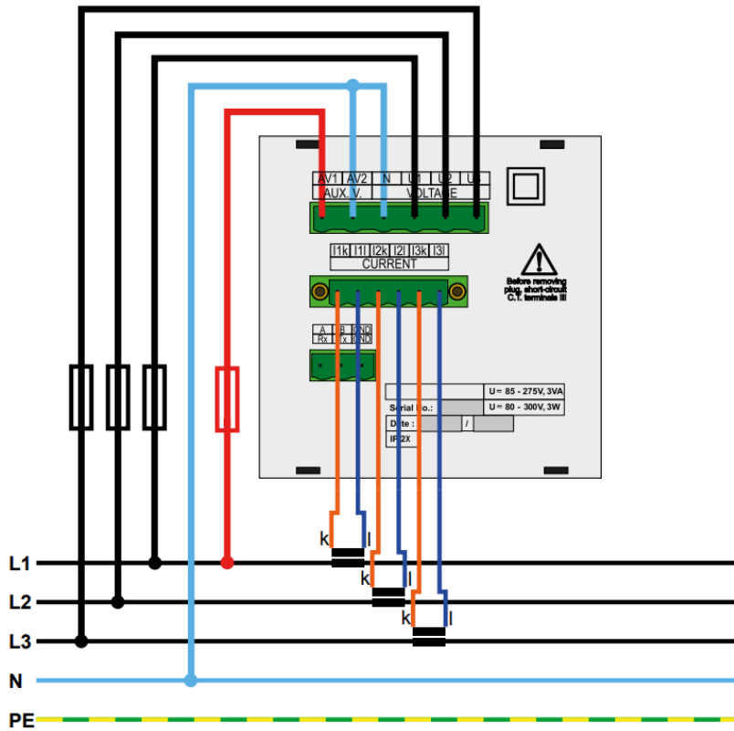
Abbildung 1: Multifunktionsmessgerät 3700X typische Installation TN-Netzwerk, Direkt-Sternschaltung („3Y“)
