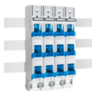
33521 NH-Sicherungs-Lasttrennleiste 250 A Größe 1, 3-polig schaltbar V-Klemme 120 mm 2
