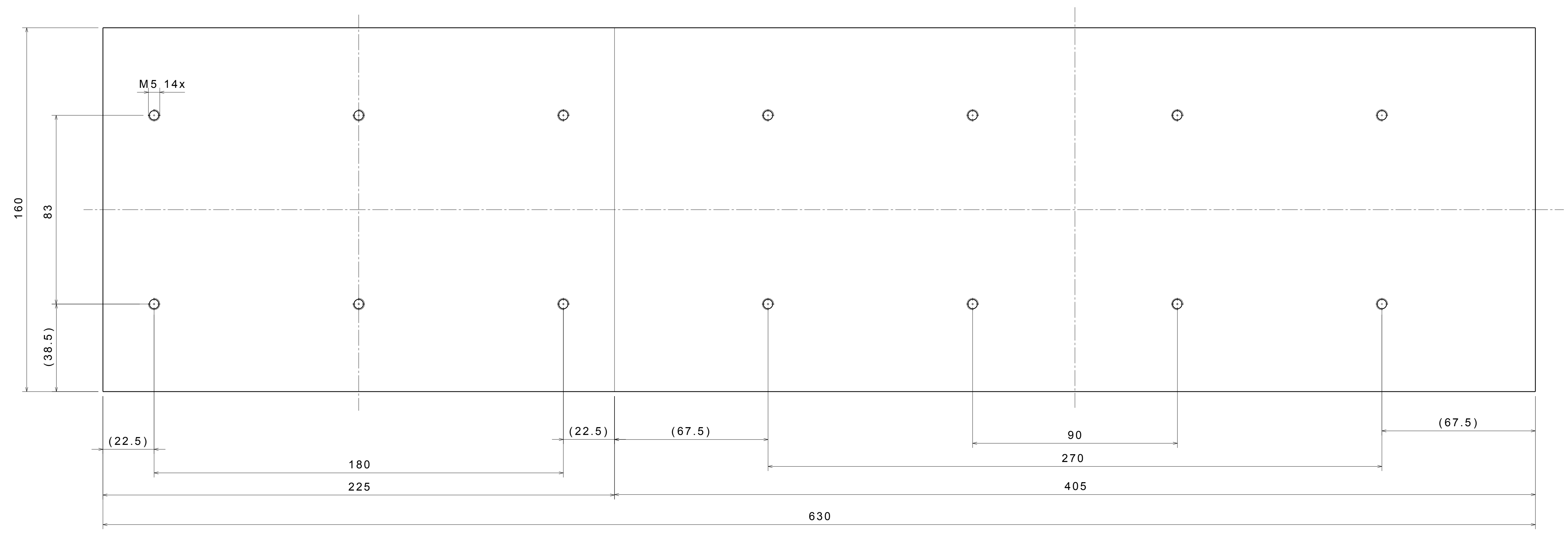
Bohrvorlage für CrossBoard® 11225A und 11405A drilling template plate for Cross Board® 11225A und 11405A
