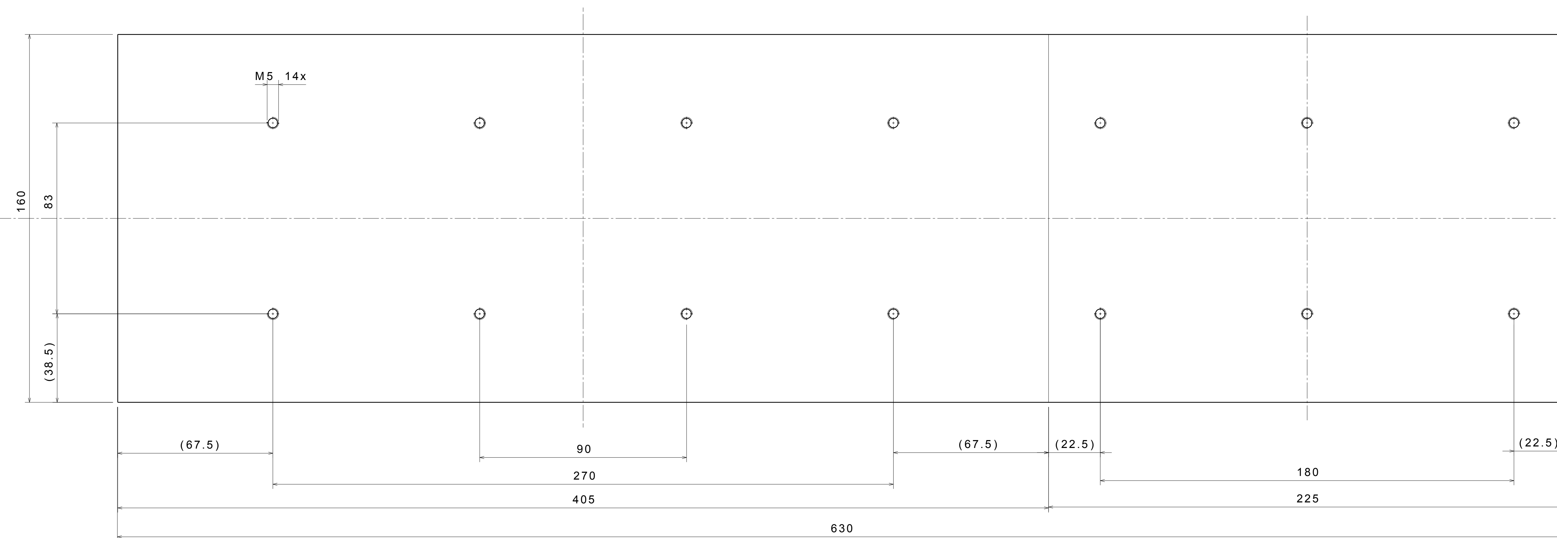
Bohrvorlage für CrossBoard® 11405A und 11225A drilling template for Cross Board® 11405A und 11225A
