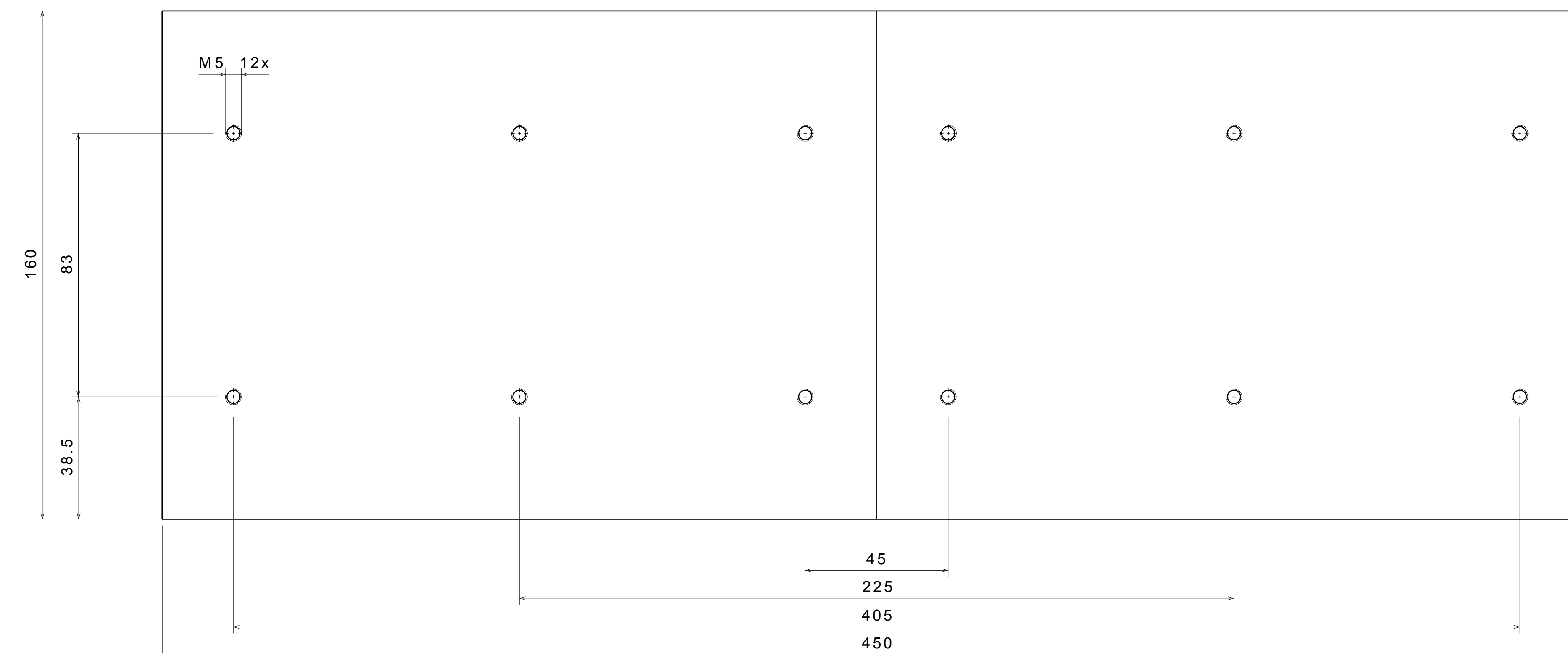
Bohrvorlage für CrossBoard® 11225A 2x drilling template plate for Cross Board® 11225A 2x
