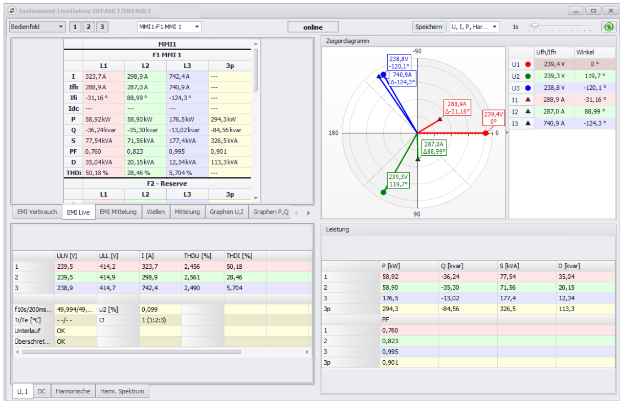
Abbildung 3: ServiceTool.Daq – LiveDaten-Fenster
