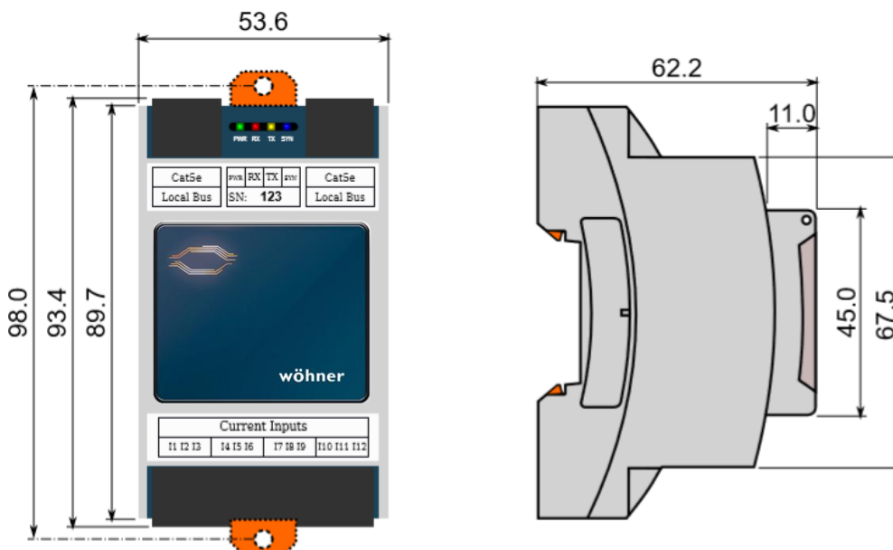
Abbildung 1: Abmessungen Stromverteilmodul 37100
