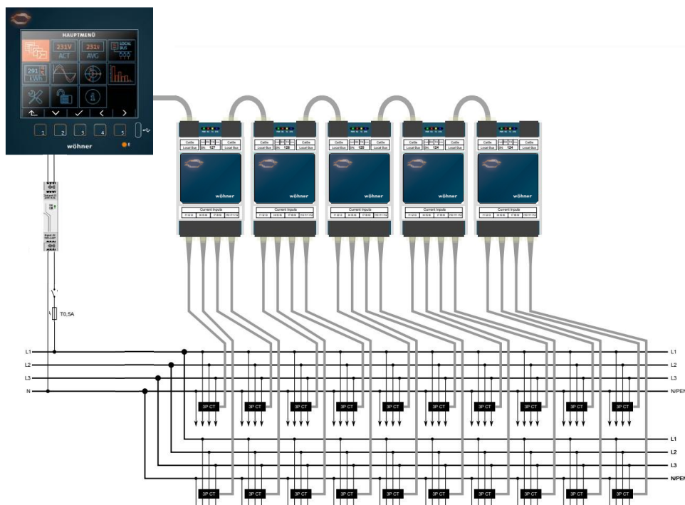
Abbildung 2: 20 Abgänge mit 5 Stromverteilmodulen 37100
