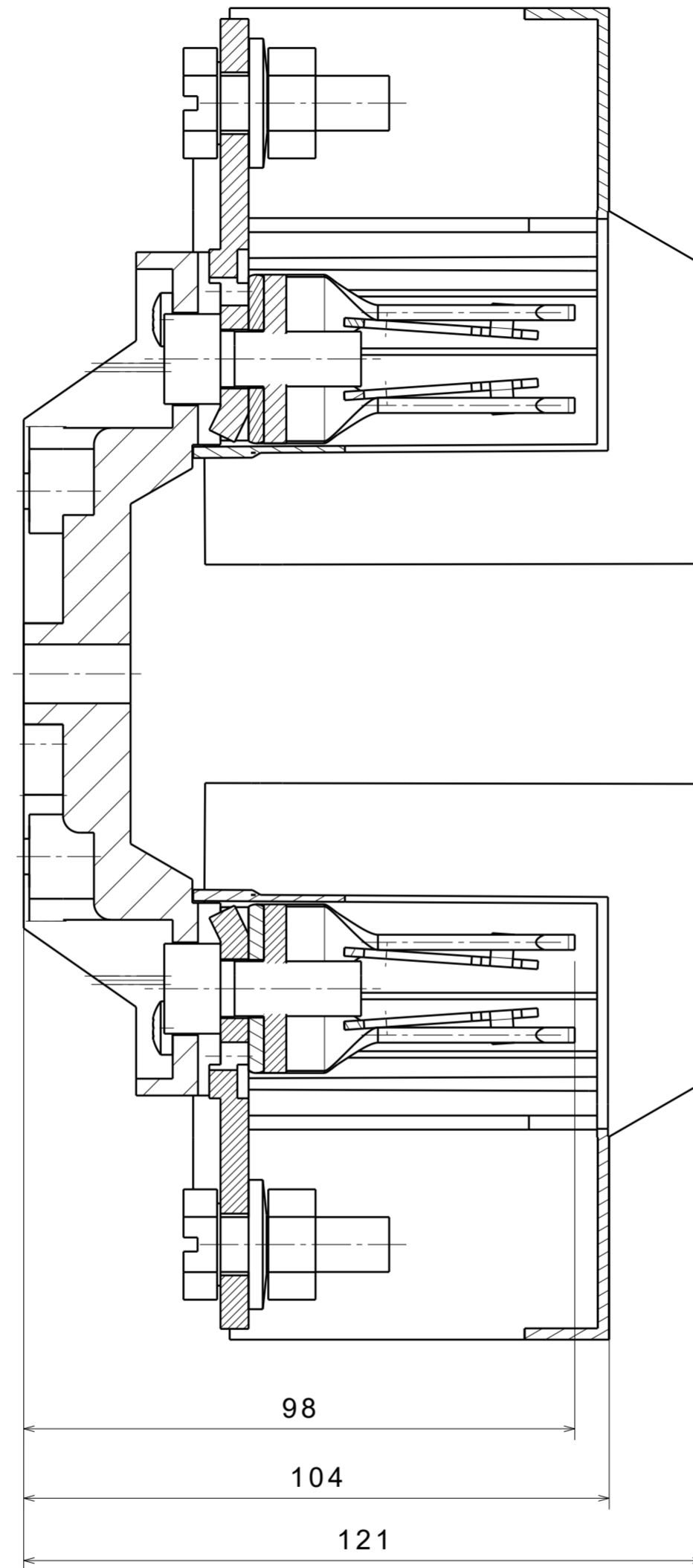
Schnittansicht A-A section view A-A Maßstab: 1:1 scale: 1:1
